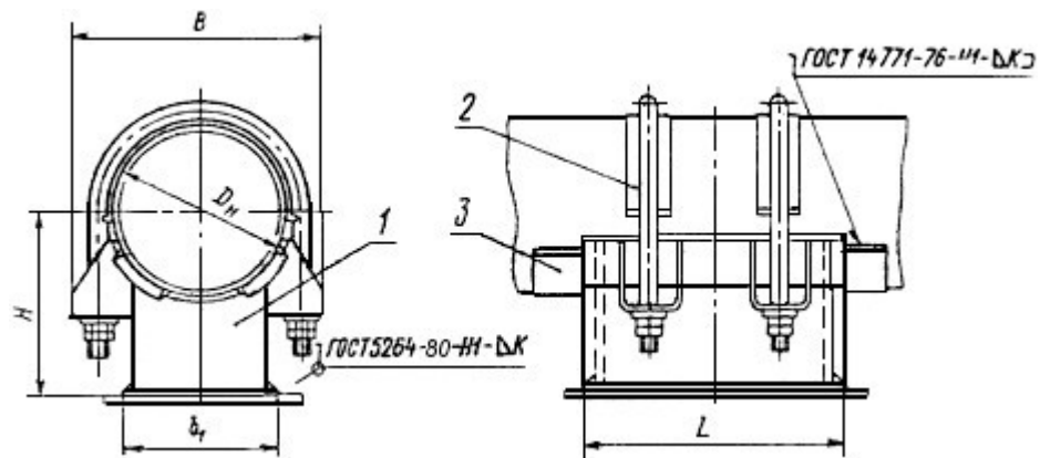
1 - опора двуххомутовая; 2 - прокладка; 3 - упор
